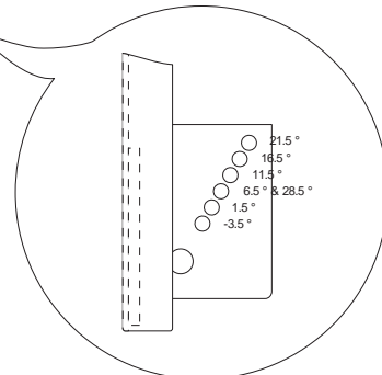
< 側面角度付 >
