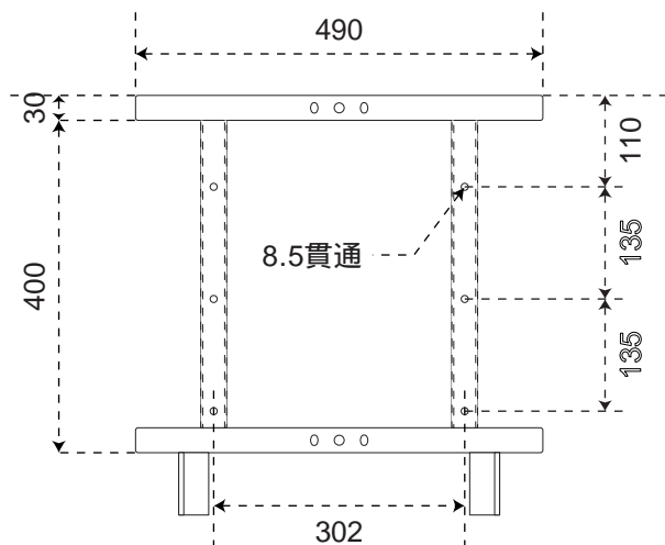
< 正面壁側部パーツ図 >
