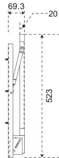
< 側面 >
