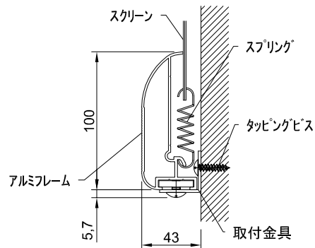
スクリーン断面詳細図
